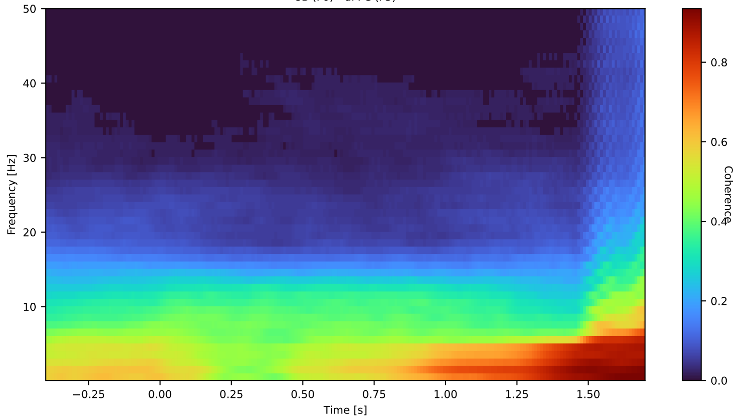
8B (F0) - dPFC (F5)
